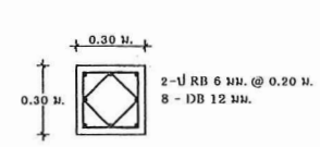
แปลนขยายฐานราก, คานคอดิน SCALE : NTS.
