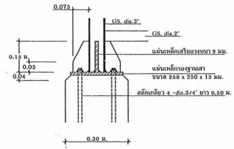
ขยายการต่อท่อเหล็กกับเสา ค.ส.ส. หมายเหตุ 1 : 10
