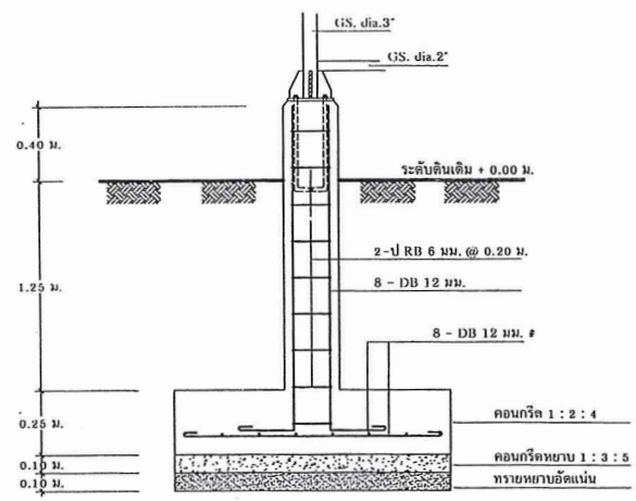
แปลนขยายฐานราก หมายเหตุ 1 : 25
