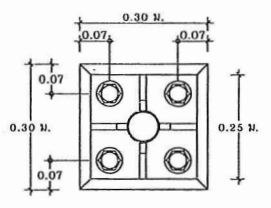
ขยายการต่อท่อเหล็กกับเสา ค.ส.ส. หมายเหตุ 1 : 10
