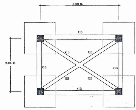
แปลนฐานราก คานคอดิน หมายเหตุ 1 : 50
