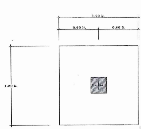
แปลนขยายฐานราก หมายเหตุ 1 : 25
