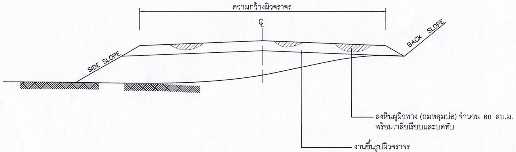
รูปตัดตามขวาง
