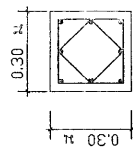
ขยายเสา มาตราส่วน 1 : 20
