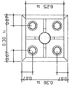
ขยายการต่อเหล็กกับเสา ค.ส.ล. มาตราส่วน 1 : 10
