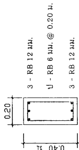
ขยายคาน GB มาตราส่วน 1 : 30
