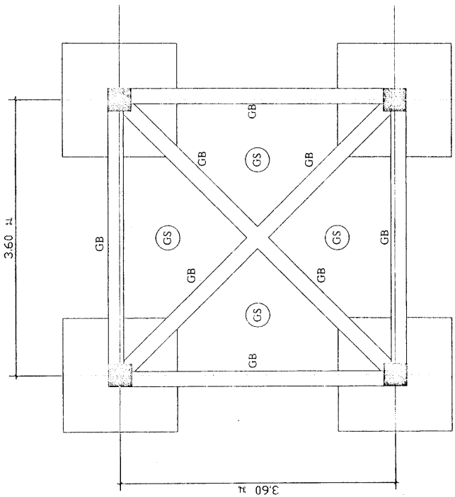
แปลนฐานราก คานคอดิน มาตราส่วน 1 : 30
